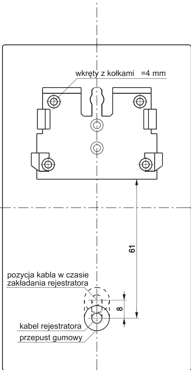
Szablon do trasowania otworów obudowy BB01
